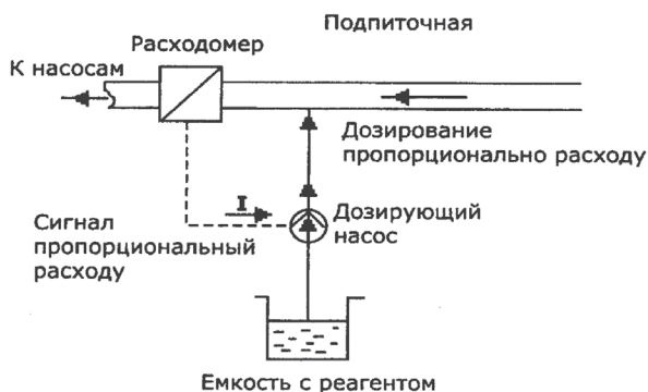
Рис.1. Типовая схема дозирования
